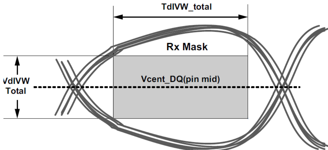
Figure 26. DQ Receiver(Rx) mask
