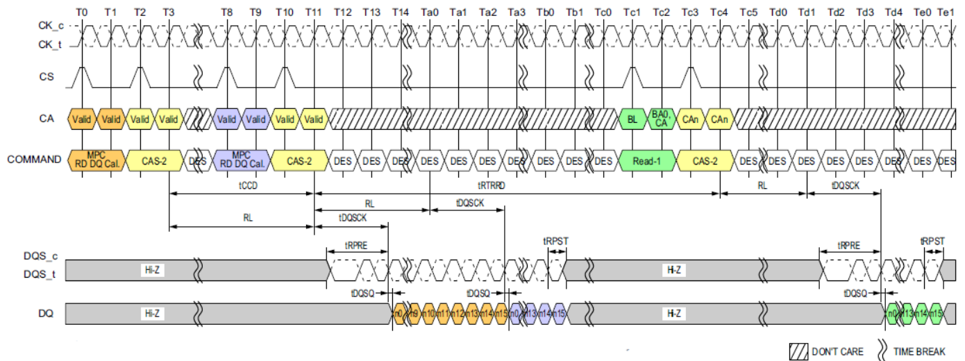
Figure 99: DQ Read Training Timing: Read DQ Cal. to Read DQ Cal. / Read
